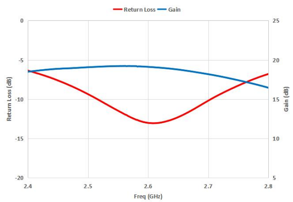
S-Parameter
