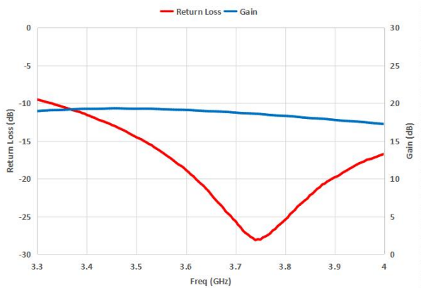
S-Parameter
